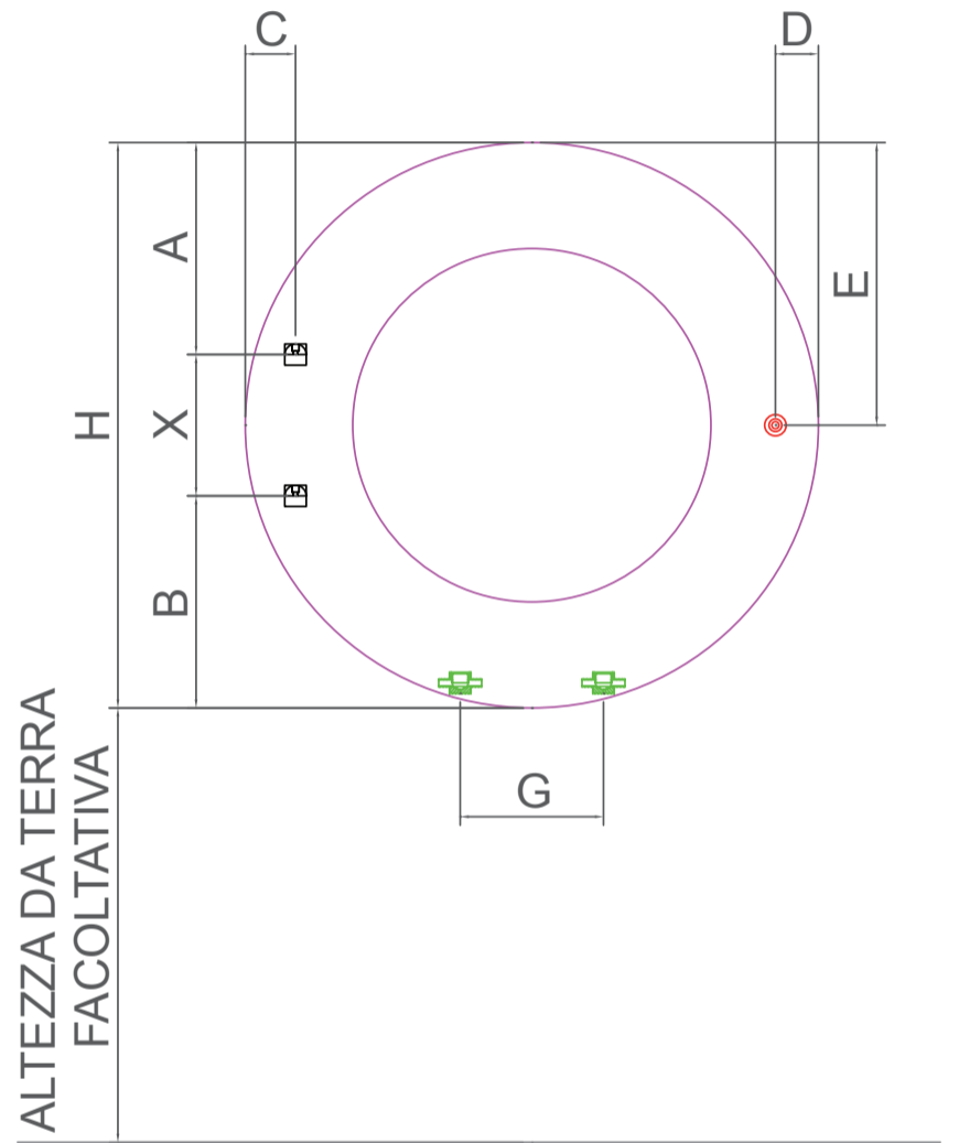
Vista frontale radiatore
